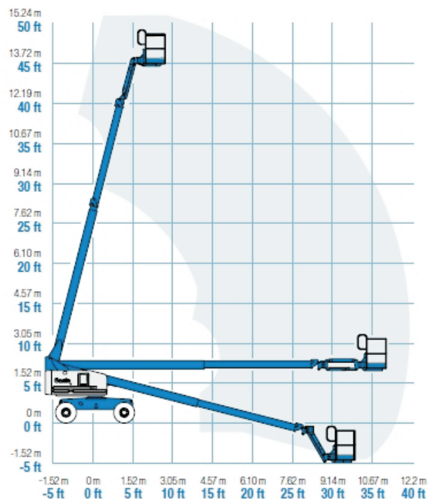
Arbeitsdiagramm S-45 / S-45 TraX
